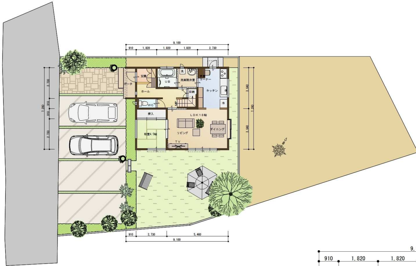
配置図・1階プラン
