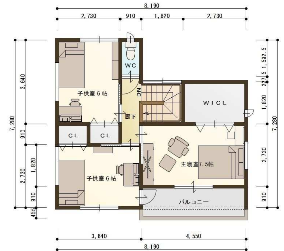
2階プラン
